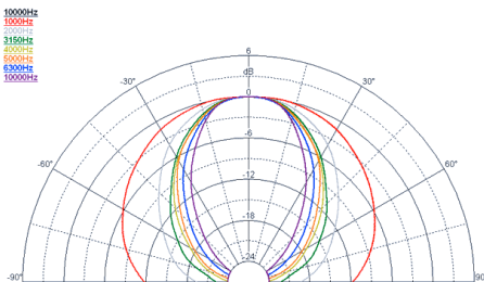
ПОЛЯРНЫЙ ГРАФИК ВЕРТИКАЛЬНОЙ НАПРАВЛЕННОСТИ
